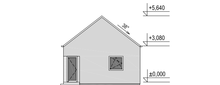
POHLED 2 M 1:200
