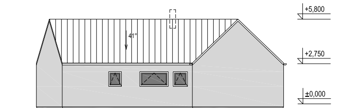
POHLED 2 M 1:250
