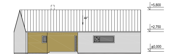
POHLED 3 M 1:250
