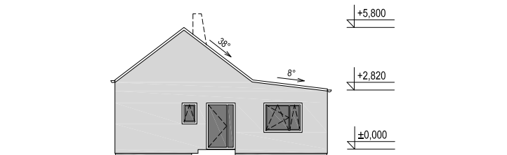
POHLED 1 M 1:250
