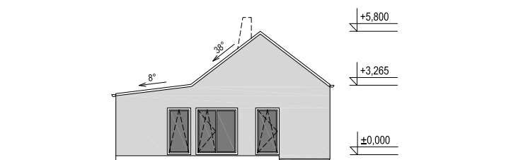
POHLED 3 M 1:250
